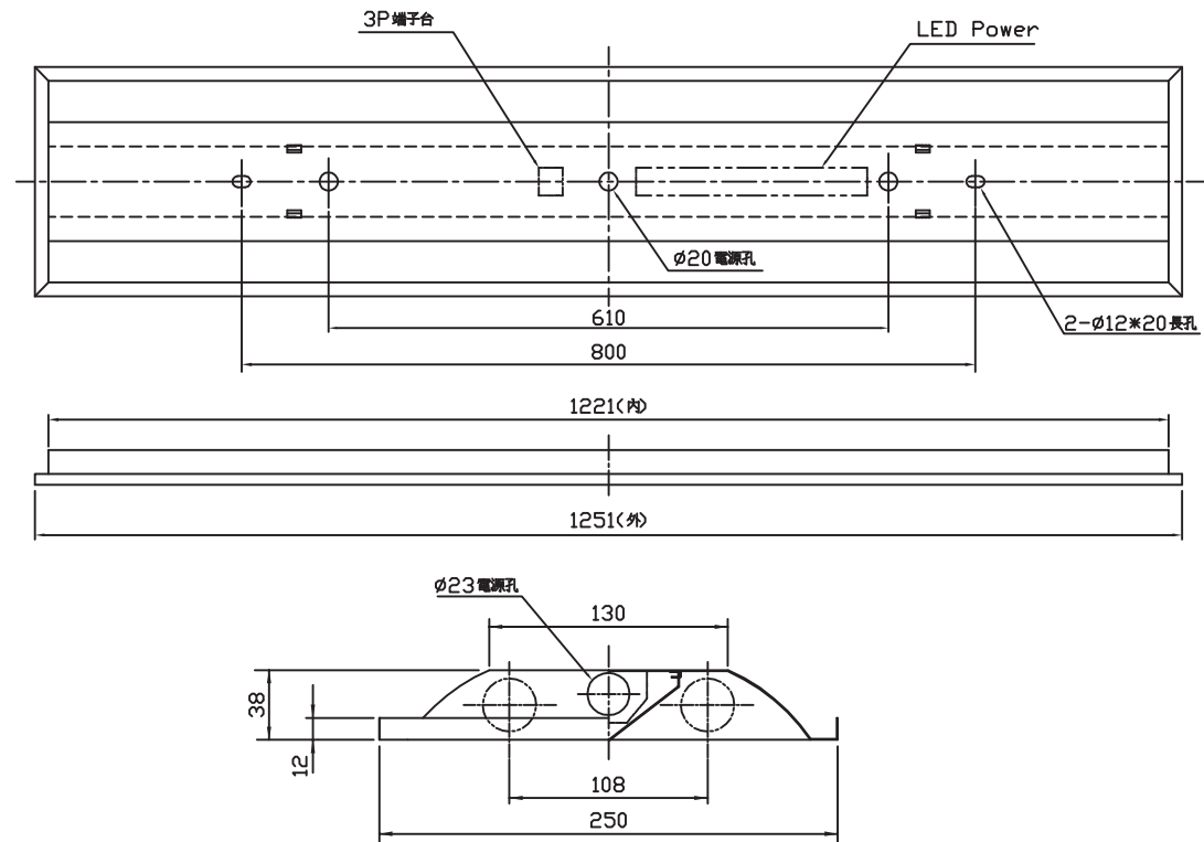
端視圖 S:2/1
